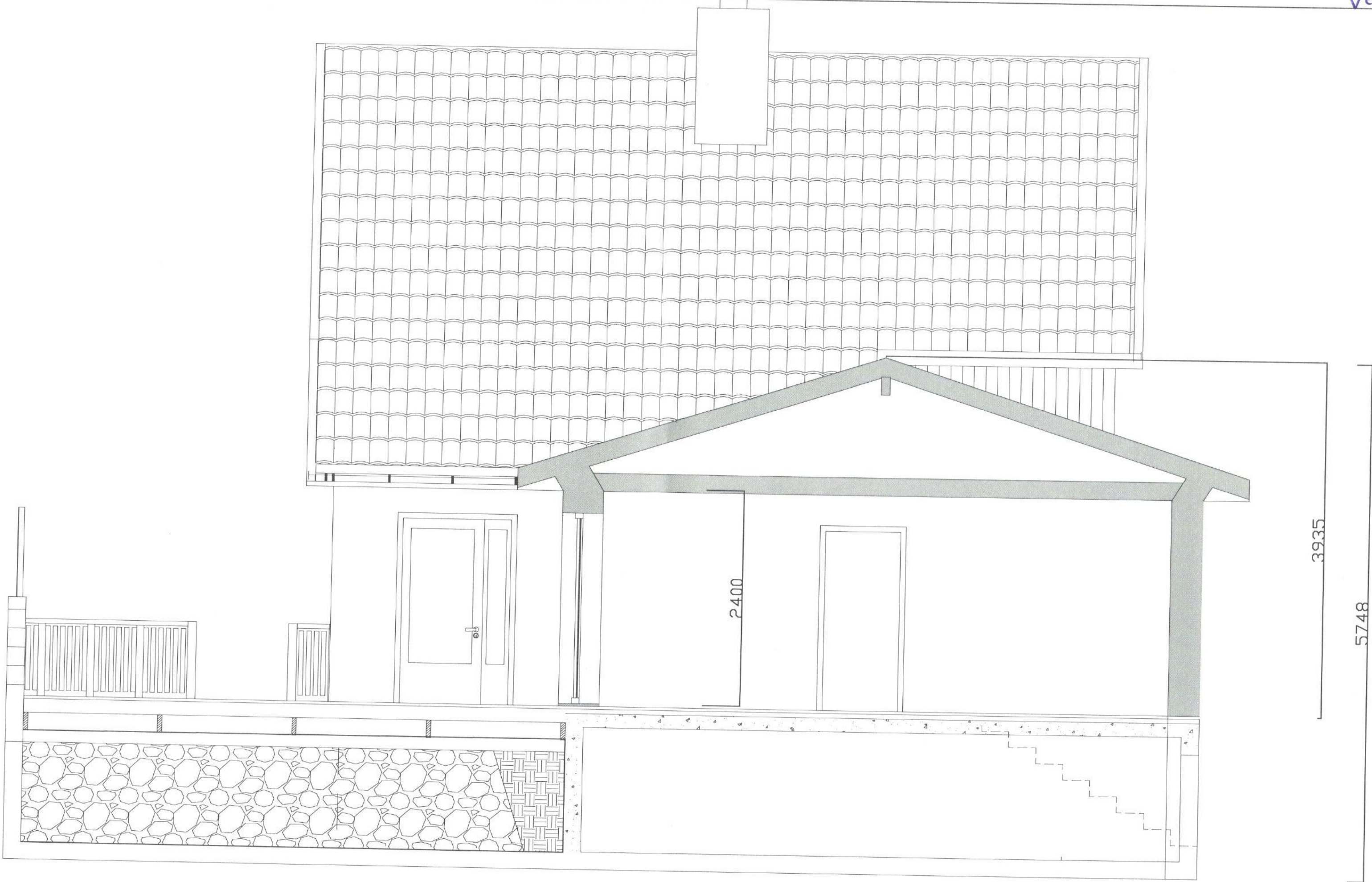
SNITT A-A
